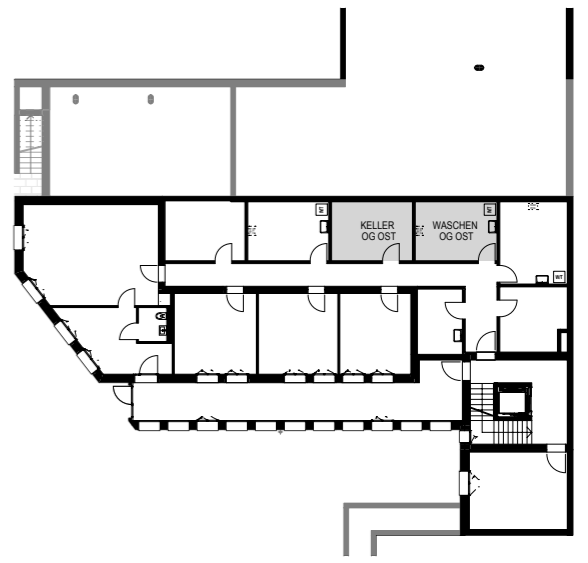
SOCKELGESCHOSS 1:400
