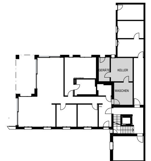
GARTENGESCHOSS 1:400
