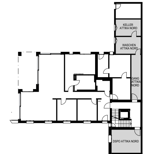
GARTENGESCHOSS 1:400
