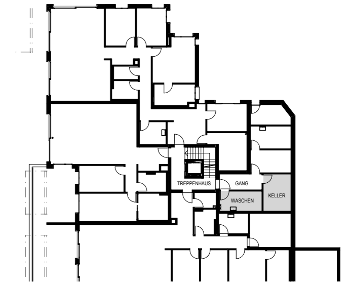
GARTENGESCHOSS 1:400
