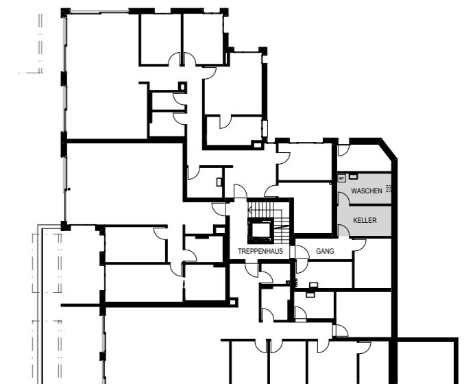
GARTENGESCHOSS 1:400
