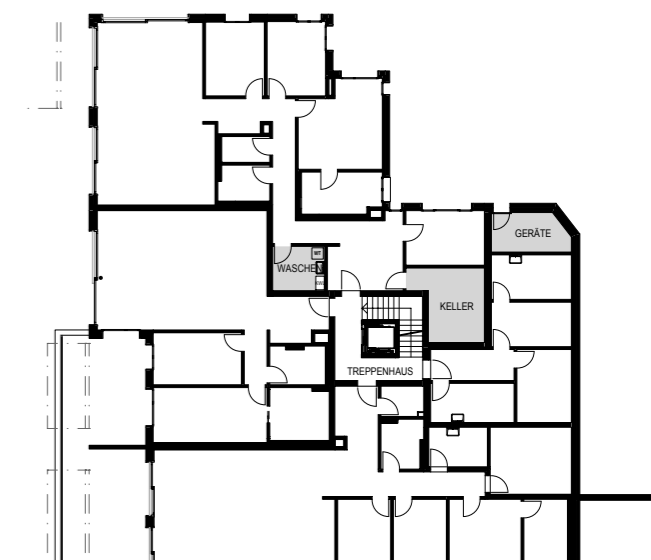
GARTENGESCHOSS 1:400
