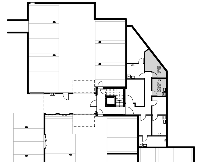
KELLERGESCHOSS 1:400
