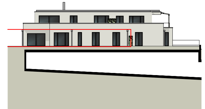
SÜDFASSADE 1:400
