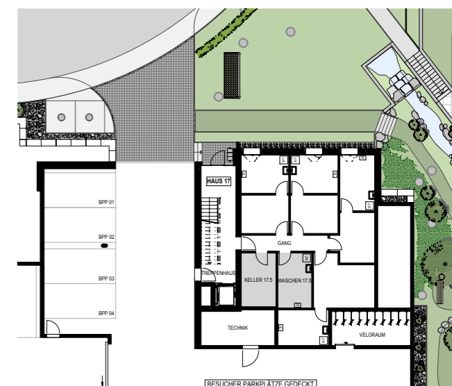
UNTERGESCHOSS 1:400
