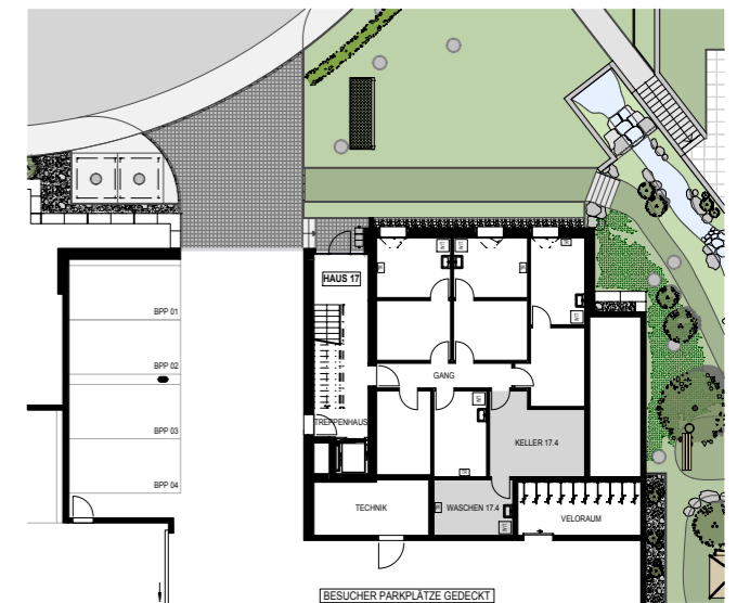
UNTERGESCHOSS 1:400
