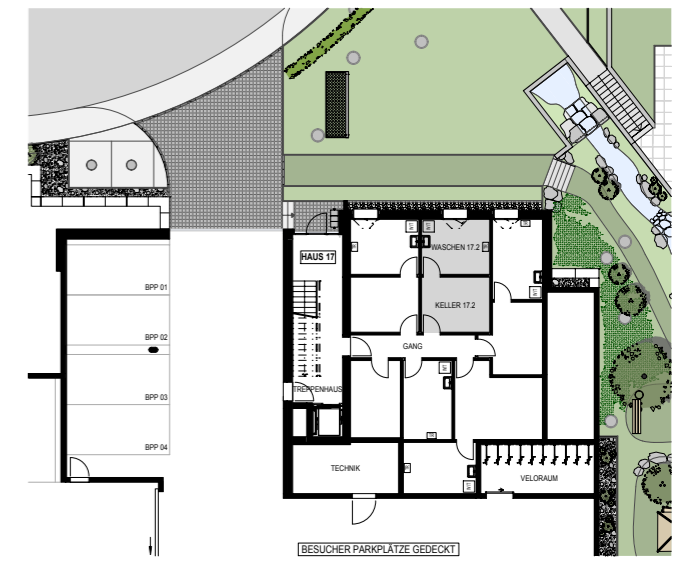
UNTERGESCHOSS 1:400
